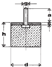
SERIE P pedino con vite filettata SERIES P Footing with upper screw
